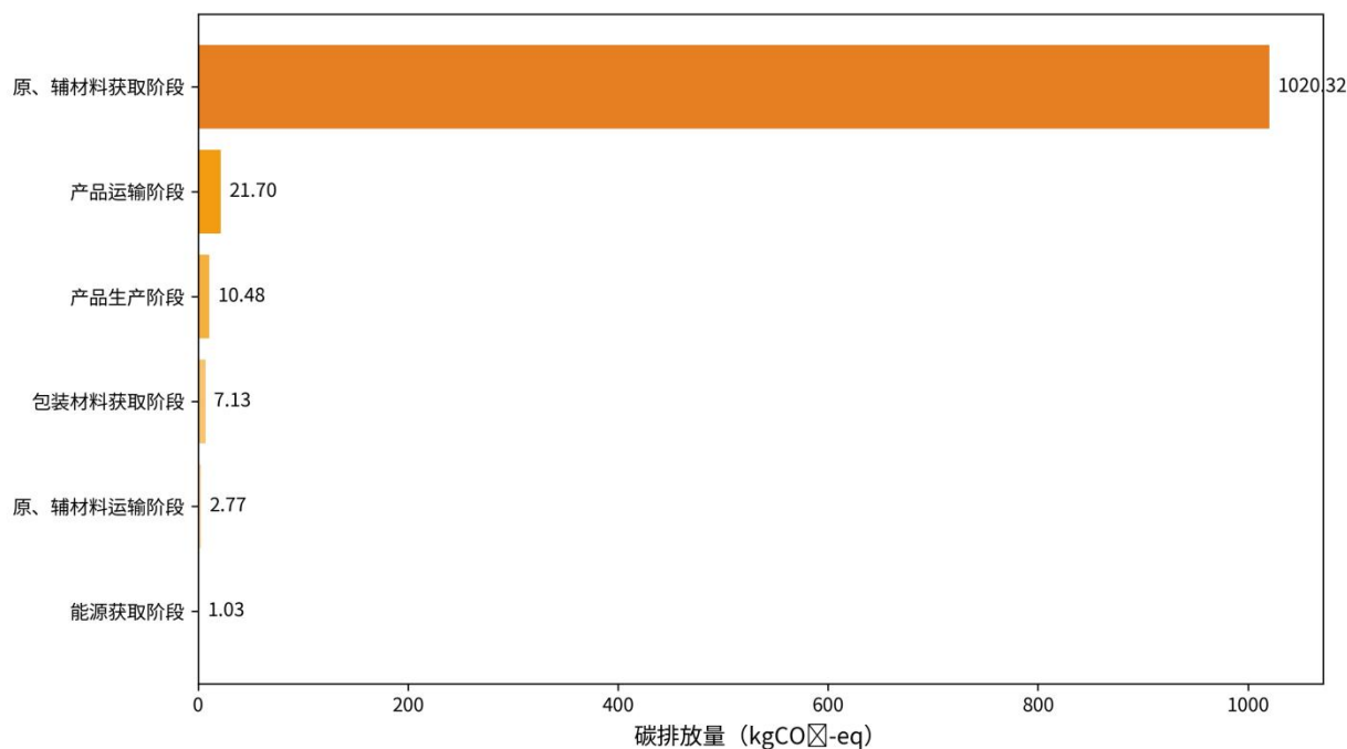
HRT-ZHJZJ-01综合集装架 各阶段碳排放量横向柱状图
