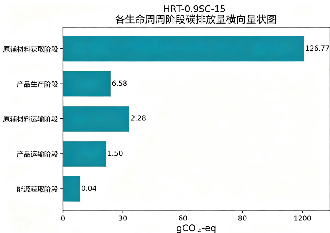
图 4 HRT-0.9SC-15 光纤活动连接器产品生命周期总图
