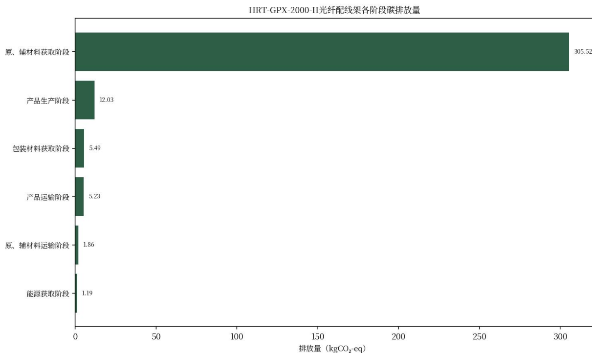
图 4 HRT-GPX-2000-II 光纤配线架产品生命周期总图
