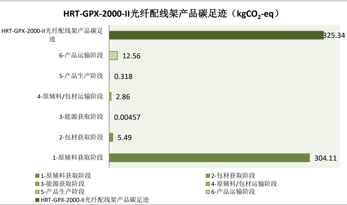
图 10 HRT-GPX-2000-II 光纤配线架产品生命周期总图
